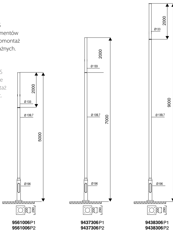
słupy stalowe / steel poles
