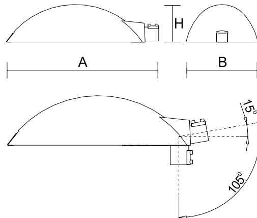
Oprawa z szybą / Luminaire with glass
