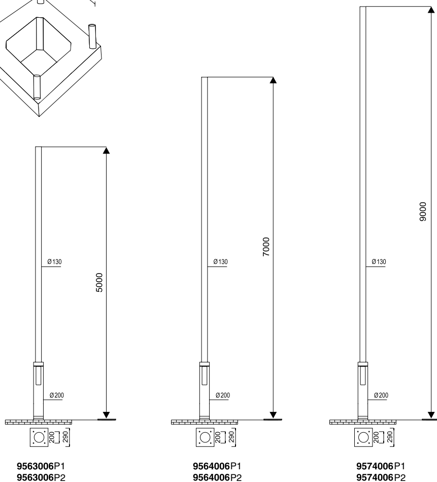
słupy aluminiowe / aluminium poles
